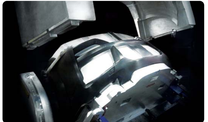
350 Tonnen Schließkraft, 30 bar Druck, 1 Sekunde Zeit: Entstehung der TECHART Magnum Frontschürze Locking force: 350 tons. Pressure: 30 bar. Injection time: 1 second. The birth of a TECHART Magnum apron
